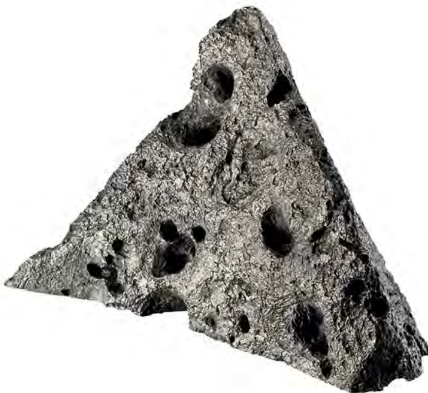
Opavský meteorit.
