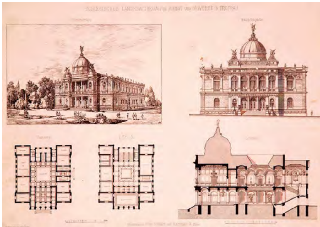
Plany Głównego Budynku Ekspozycyjnego
